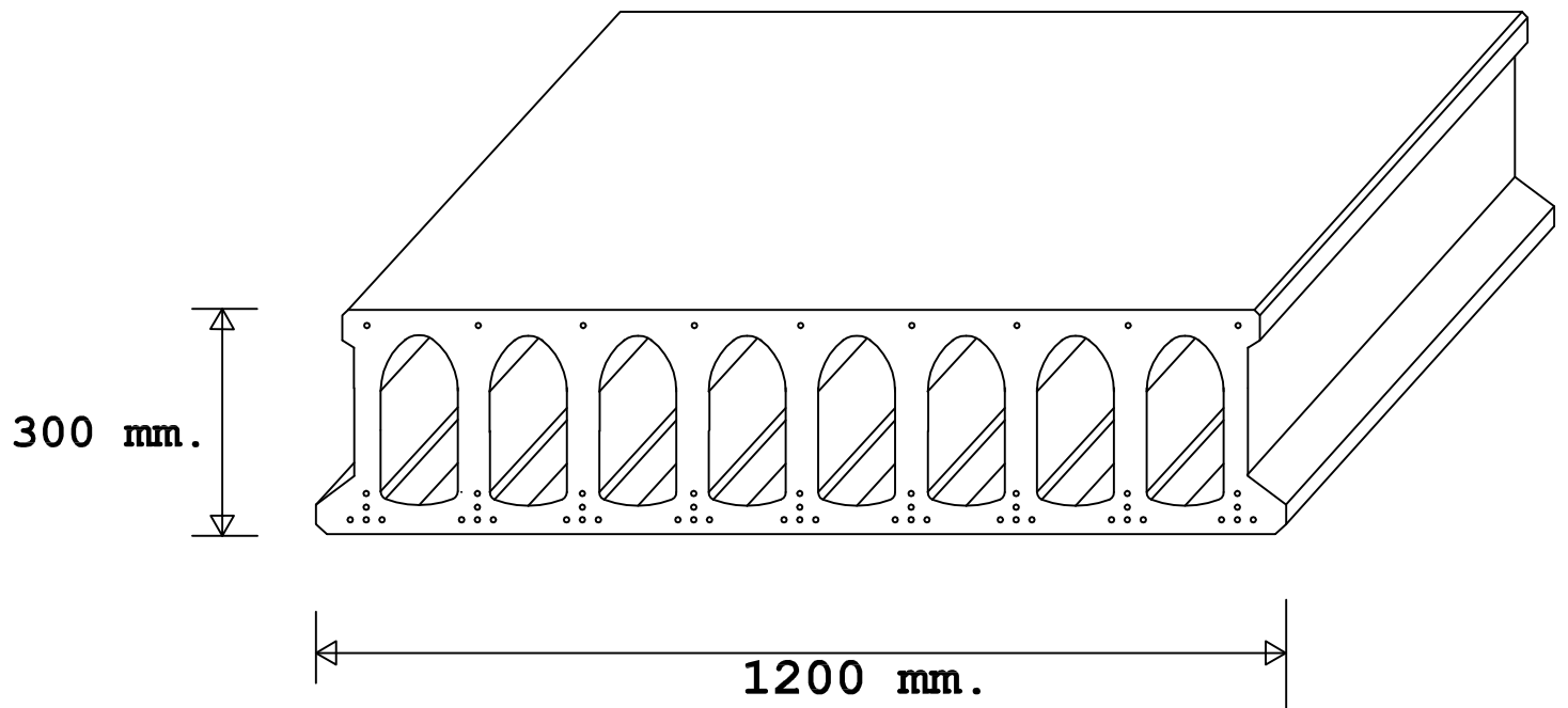
PLACA ALVEOLAR PARA FORJADO DE 300 MM. DE CANTO PESO DE LA SECCION POR METRO CUADRADO 377 KG.
