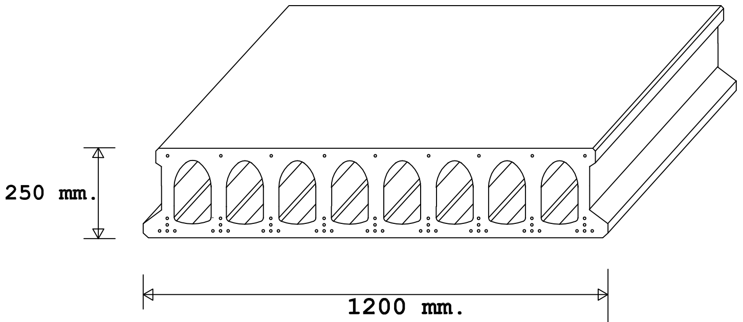
PLACA ALVEOLAR PARA FORJADO DE 250 MM. DE CANTO PESO DE LA SECCION POR METRO CUADRADO 325 KG.
